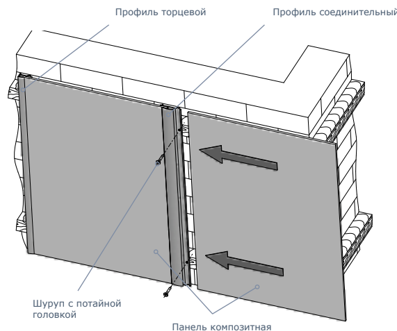
Соединительный ALUM 4011
